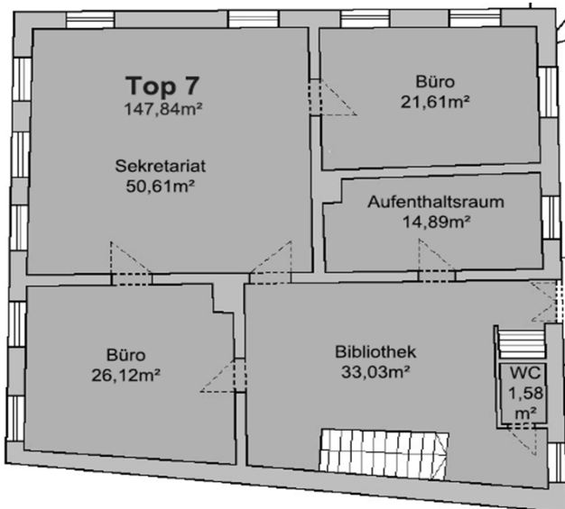
Obergeschoß
